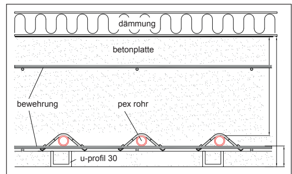
beispiel: rohrbefestigung auf der unteren bewehrung
